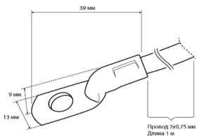
Рис. 2 Габариты датчика температуры
