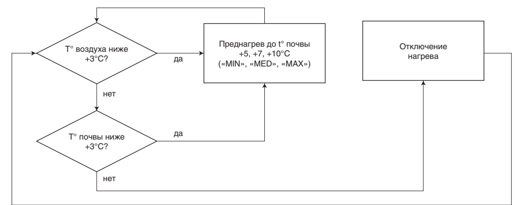
Блок-схема 4. Алгоритм работы метеостанции в режиме «MODE 03» при наличии датчиков ДТП и ДОТ
