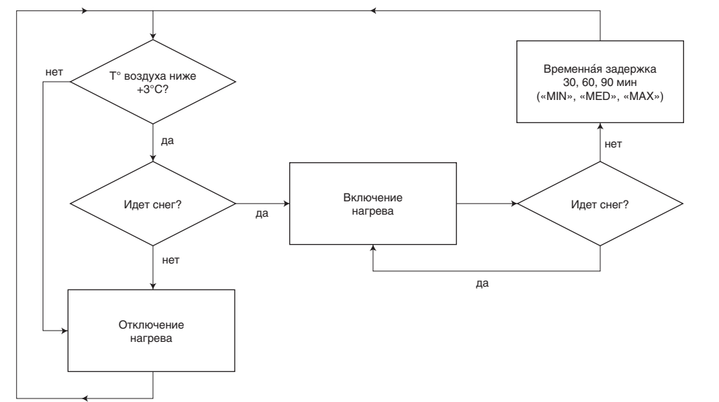
Блок-схема 2. Алгоритм работы метеостанции в режиме «MODE 02»
