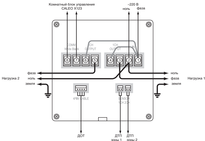
Схема 1. Электроподключение метеостанции CALEO UTH-X123 при токах коммутации меньше 15 А с учетом пусковых токов. Вид сзади: клеммы для подключения дополнительного оборудования
