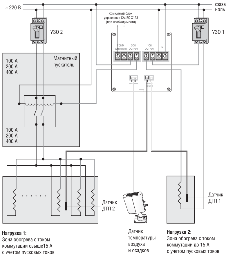
Схема 2. Электроподключение метеостанции CALEO UTH-X123 при токах коммутации больше 15 А с учетом пусковых токов
