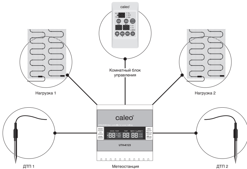
Рис. 3. Набор элементов метеостанции для режима управления «MODE 03»
