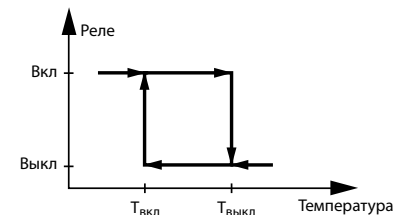
Рис. 10. Гистерезис работы.
